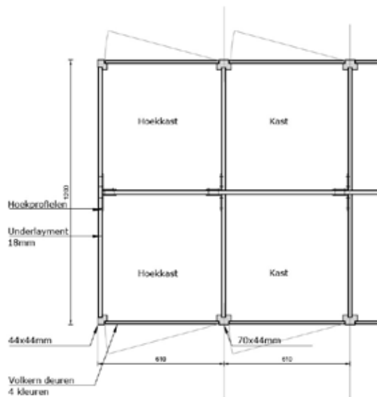
PRINCIPE OPBouw KAST 1:10
